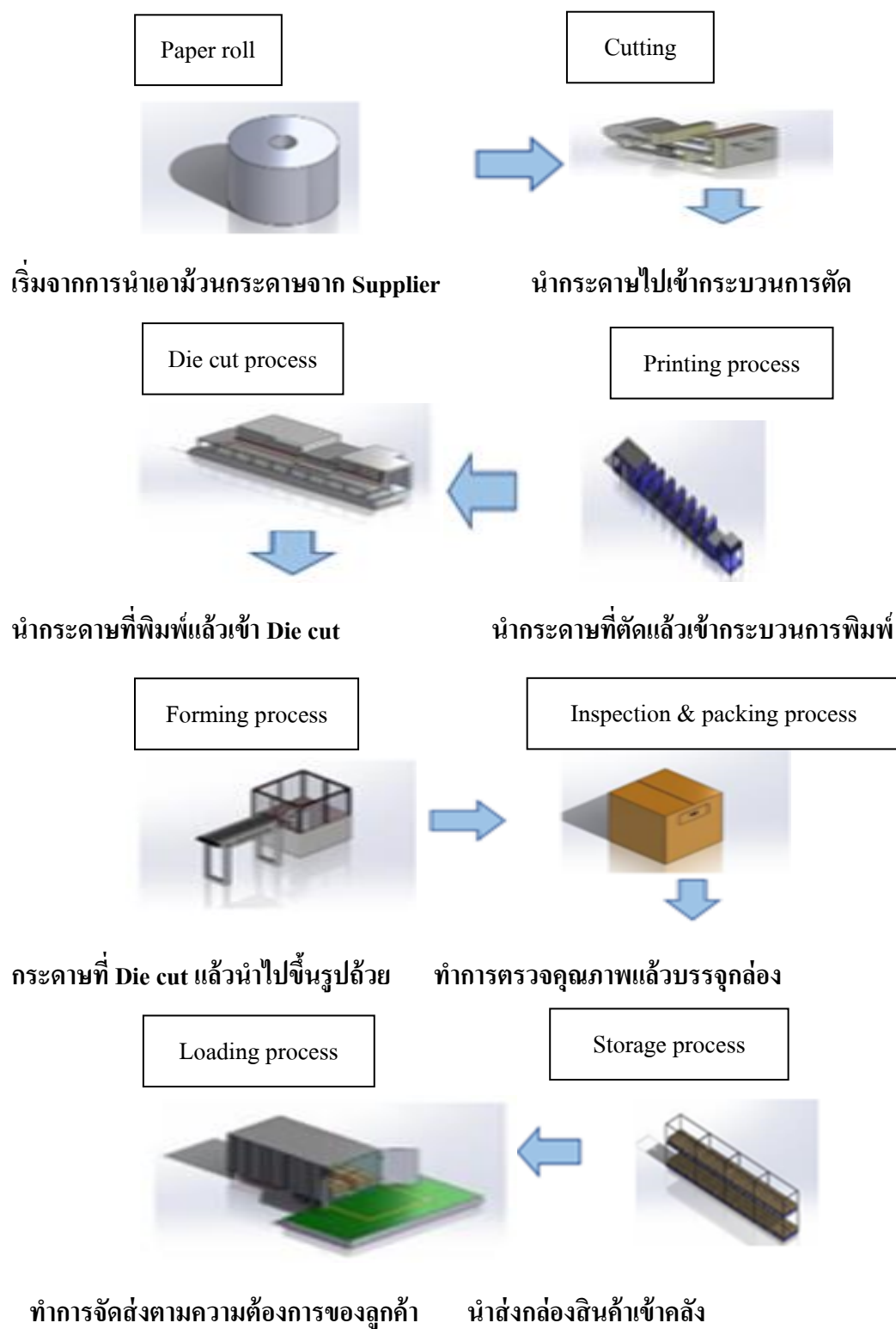
ภาพที่ 4 ฝั่งกระบวนการผลิตกระดาษ
